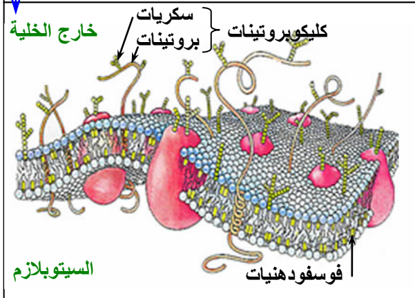
أنموذج البنية الجزيئية للغشاء السيتوبلازمي
